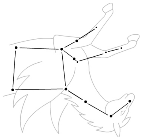
Pegasus
