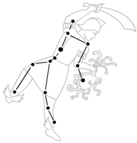
Perseus
