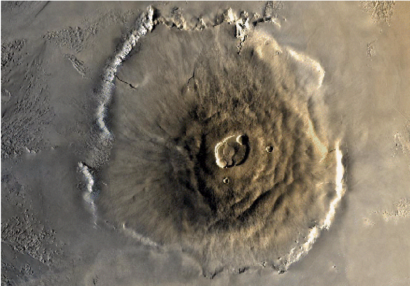
Foto: NASA, Viking Project
